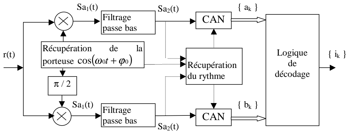
Figure 23 : Démodulateur MDP-M
