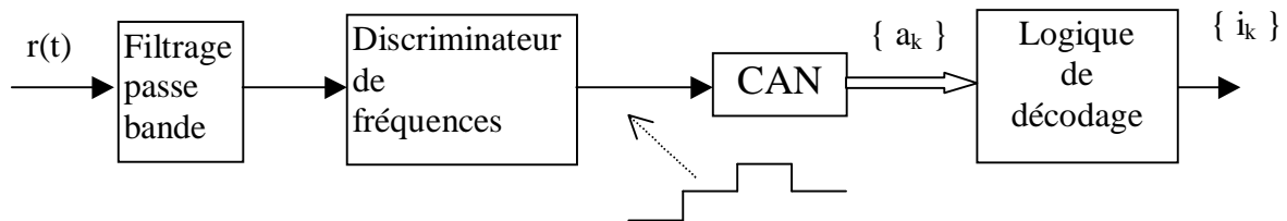
Figure 31 : Démodulateur MDF-M-PC
